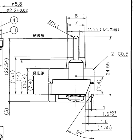
右側面図 (2/1)
